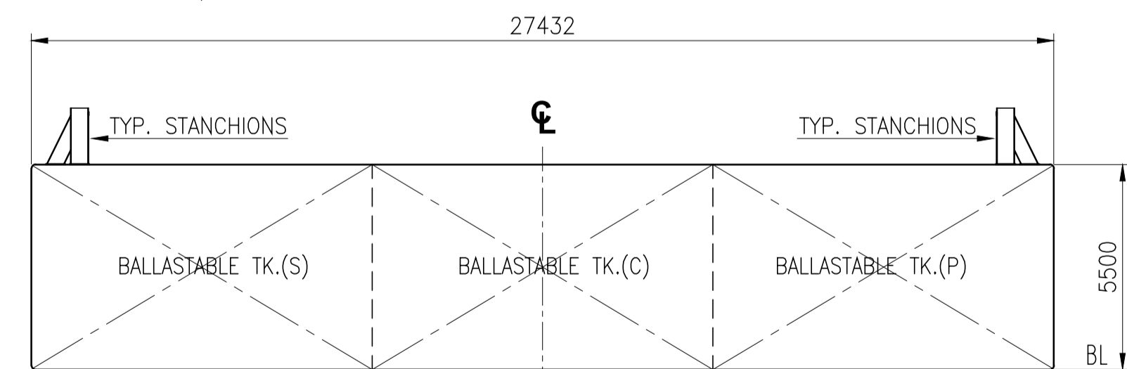
TRANSVERSE SECTION LKG. FWD / N.T.S
