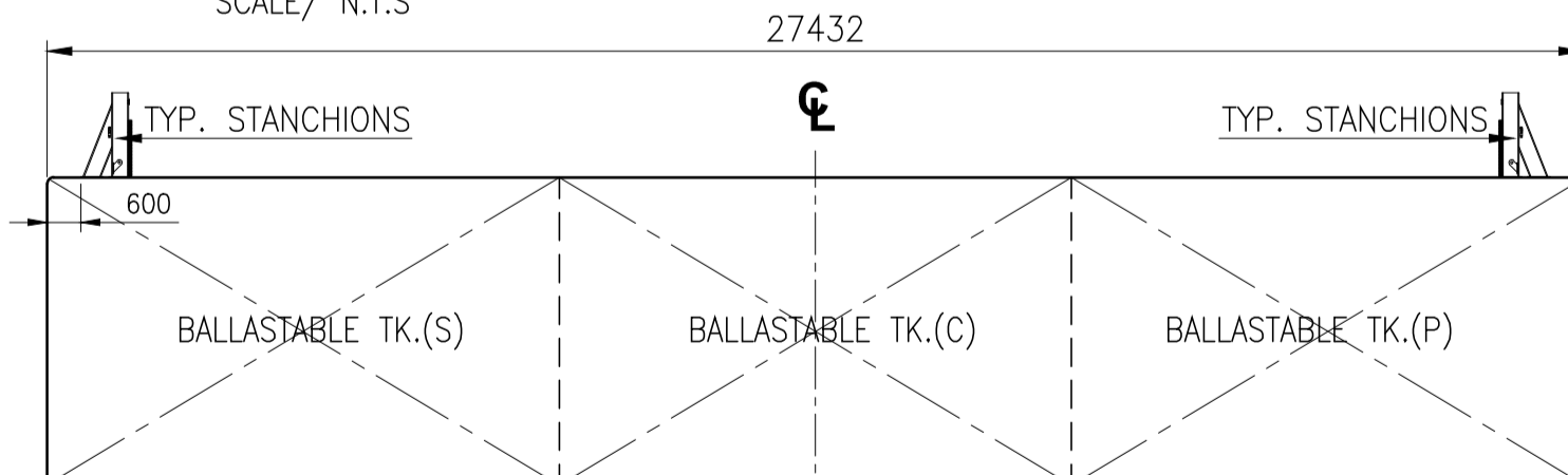
TRANSVERSE SECTION LKG. FWD / N.T.S
