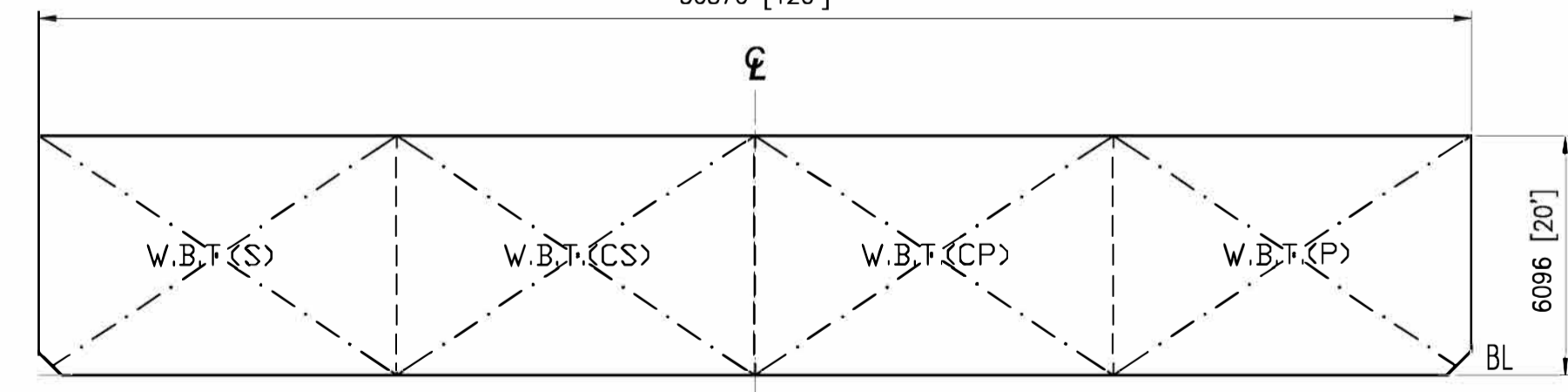
TRANSVERSE SECTION LKG. FWD / N.T.S
