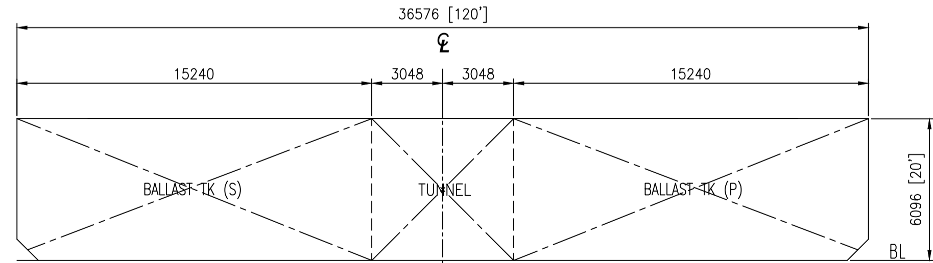
TRANSVERSE SECTION LKG. FWD / N.T.S.
